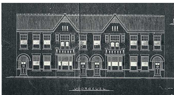
Voor- en achtergevel.
