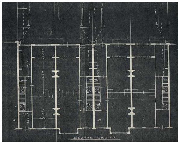
Begane grond en verdieping.
